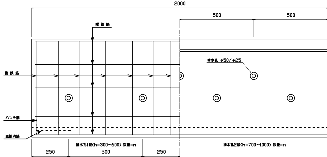
側面図
