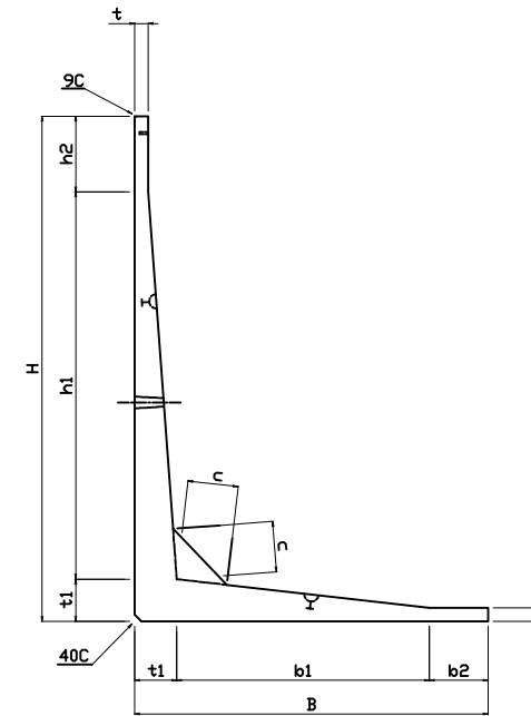
側面図
