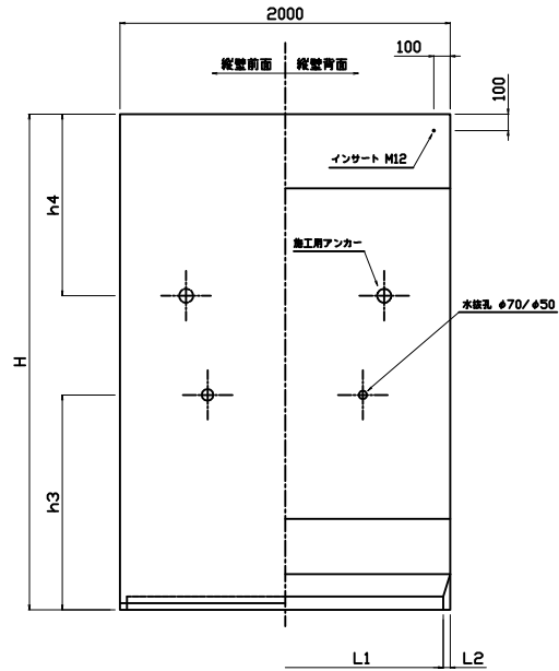
正(背)面図
